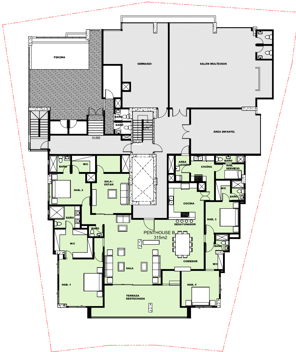
① PLANTA AMUEBLADA - NIVEL 9 1:75
