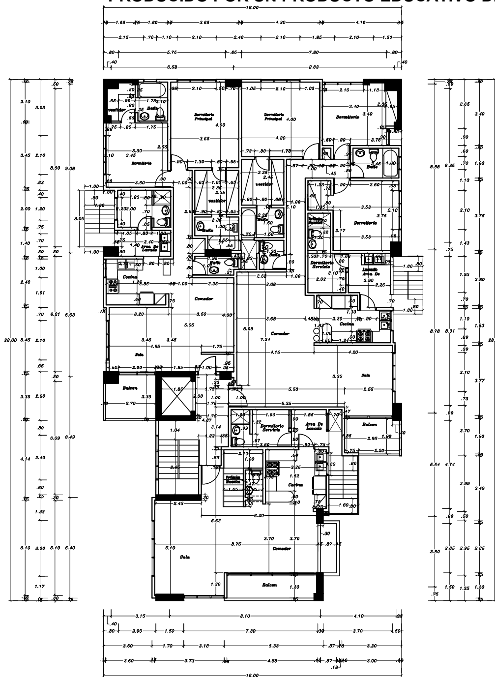
PLANTA ARQUITECTONICA 4to Y 6to NIVEL ESC. 1:150
